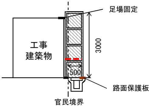
横断面図 （単位:mm）
